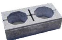
Metropol Uni 1/2 - univerzálny prvok - rezaním možno vytvoriť 2 ks polovičných - krajových prvkov - rozmery: 40 x 20 x 10 cm
