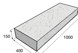
Schod VERTO 1
